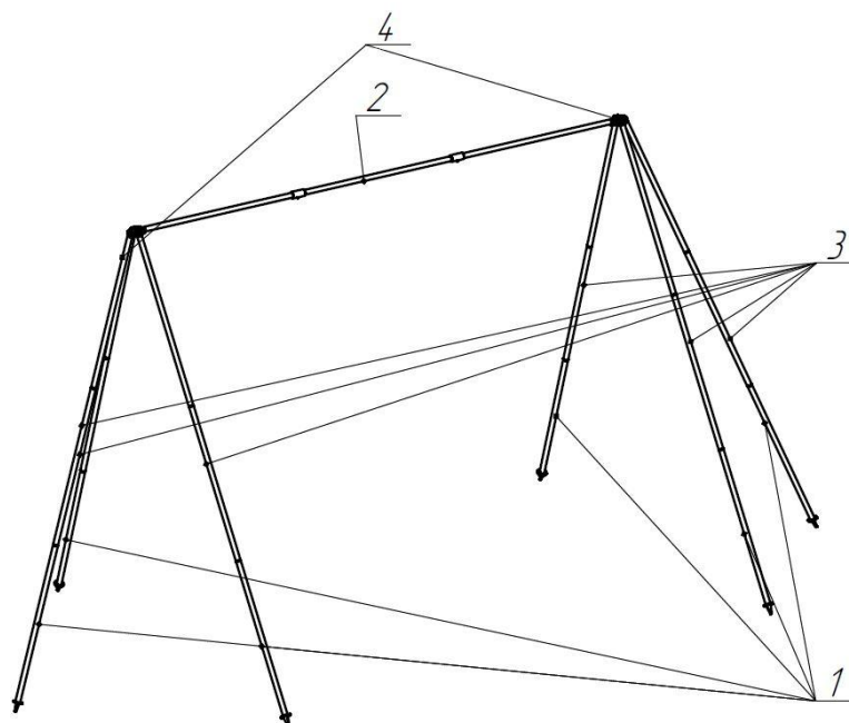
Рис. 2 Палатка монтажная ПМК. Каркас без тента, вид сбоку.
